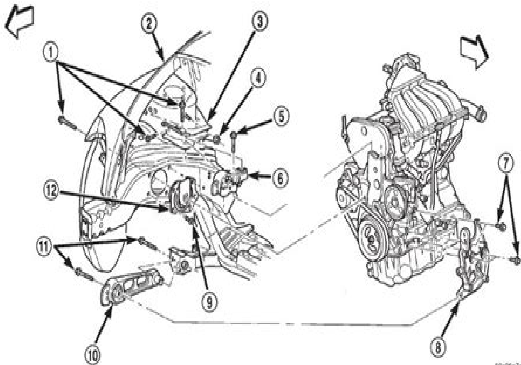
Fig. 8 Montaje del motor—Lado derecho
